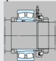
(d) Removal by use of locknuts
